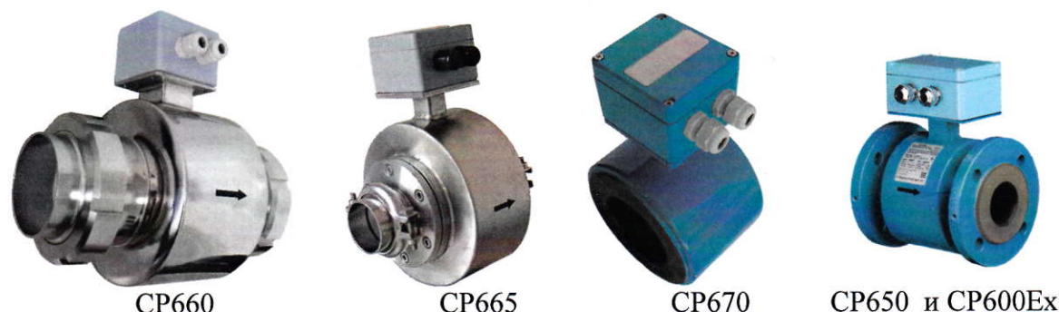
Рисунок 1 - Общий вид датчиков расходомеров электромагнитных MERA EFM/EFM Ex
